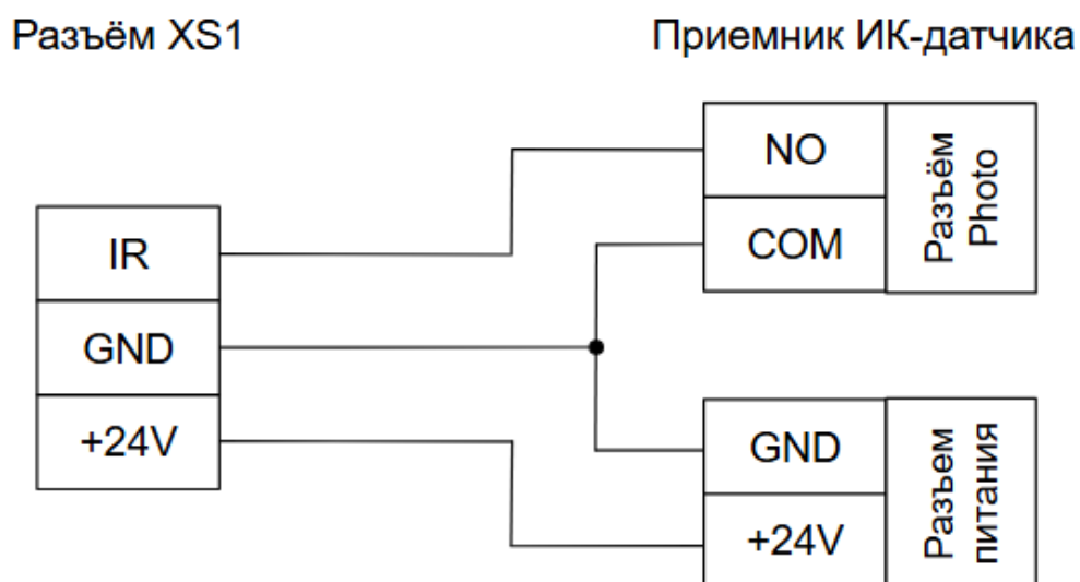
Рисунок 29. Схема подключения фотоэлектрических датчиков
