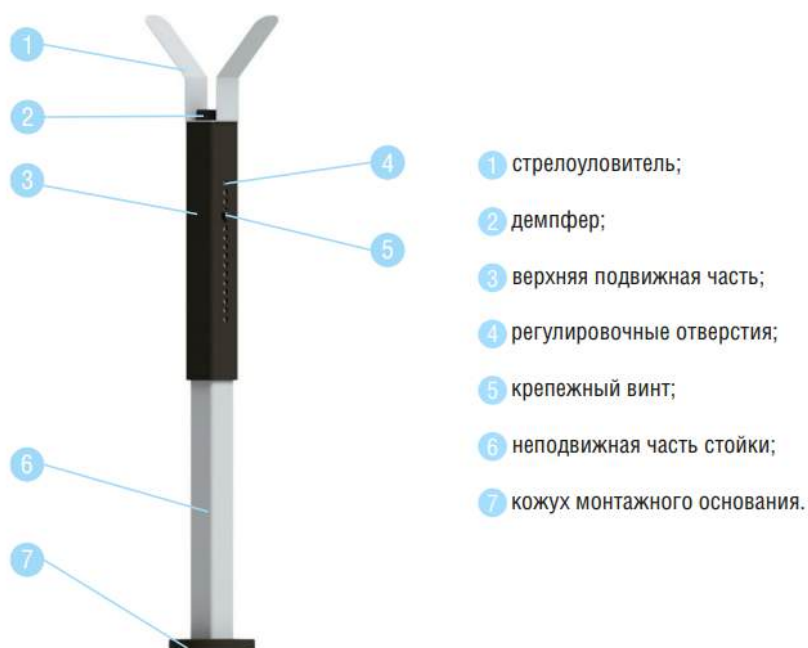
Рисунок 24. Опора стрелы
