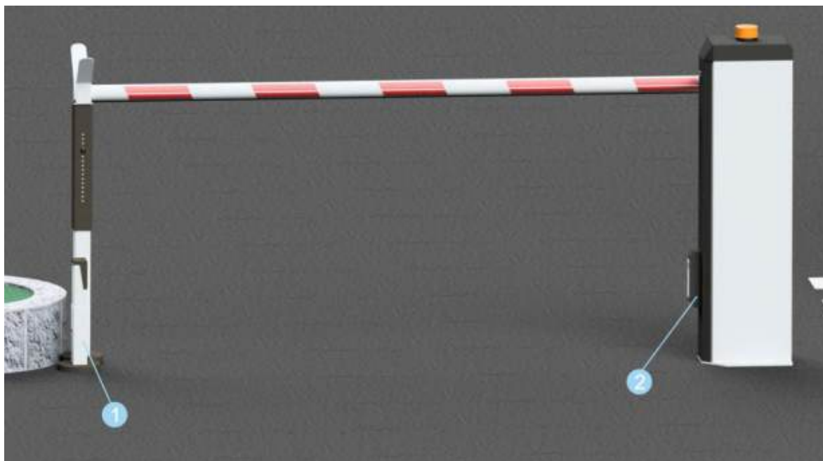
Рисунок 16. Схема расположения фотоэлементов
